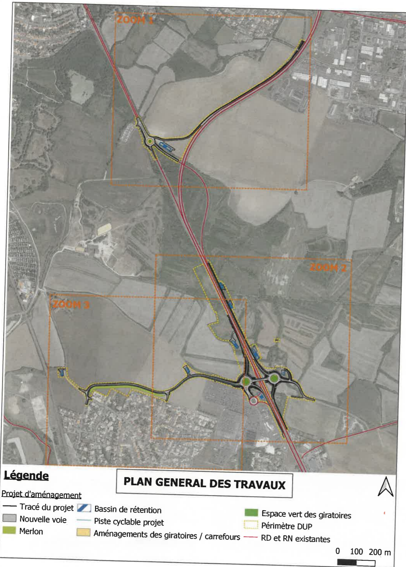
Figure 1 : Plan général des travaux et localisation des zooms
